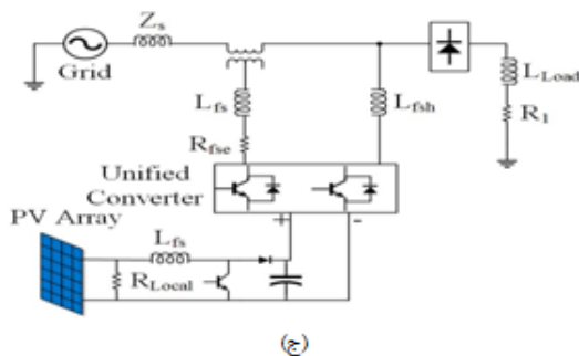
شکل (۴): سیستم تحت بررسی، الف) سناریوی اول، ب) سناریوی دوم و ج) سناریوی سوم
