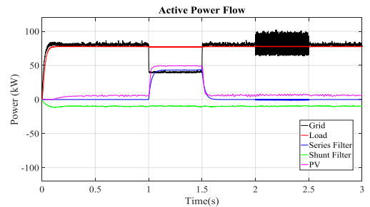
شکل (۱۷): نحوه شارش توان اکتیو در سناریوی دوم
