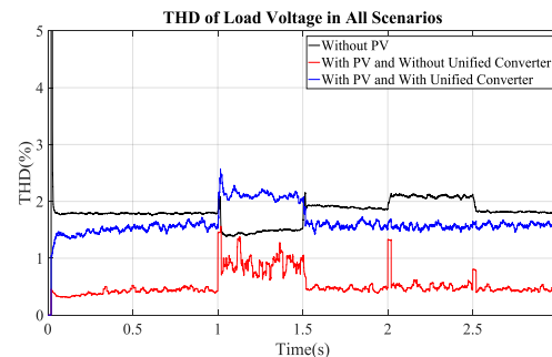
شکل (۲۱): مقایسه محتوای هارمونیک ولتاژ بار در سه سناریو
