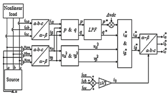
شکل (۶): تئوری p-q لحظه‌ای برای کنترل فیلتر اکتیو موازی [۱۳]
