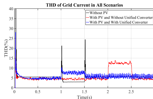
شکل (۲۲): مقایسه محتوای هارمونیک جریان منبع در سه سناریو
