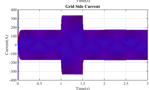
شکل (۹): نتایج شبیه‌سازی سناریوی اول
